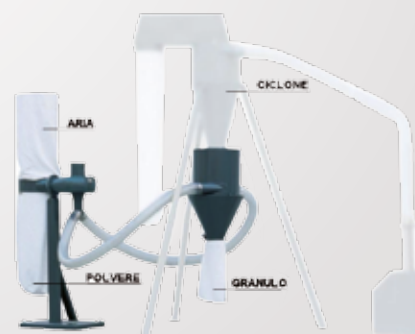
Dust separator. Separatore di polvere.
