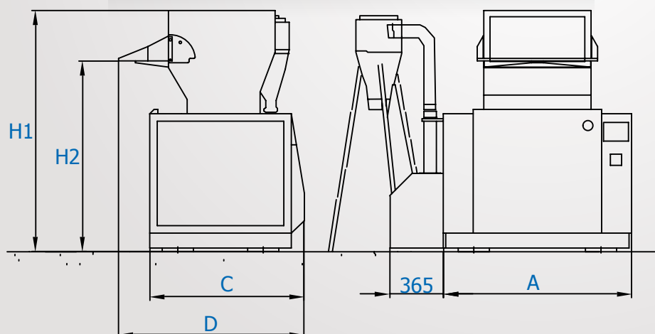
Dust separator. Separatore di polvere.
